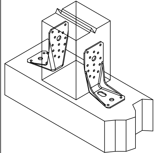
Para kątowników na połączenie
