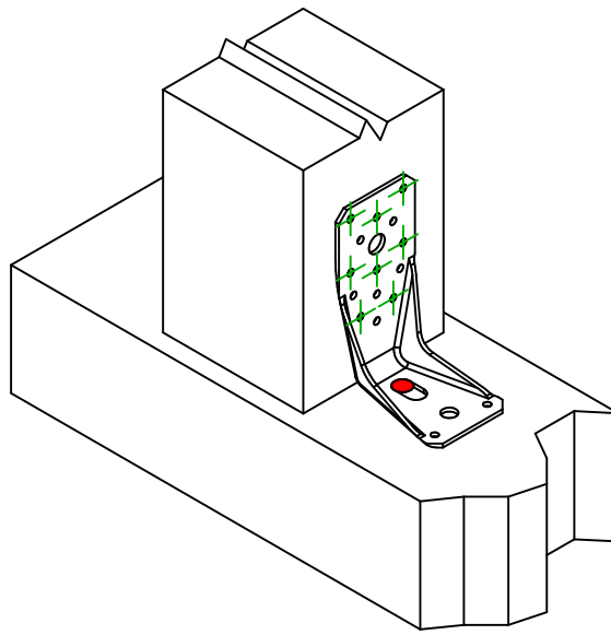
Jeden kątownik na połączenie
